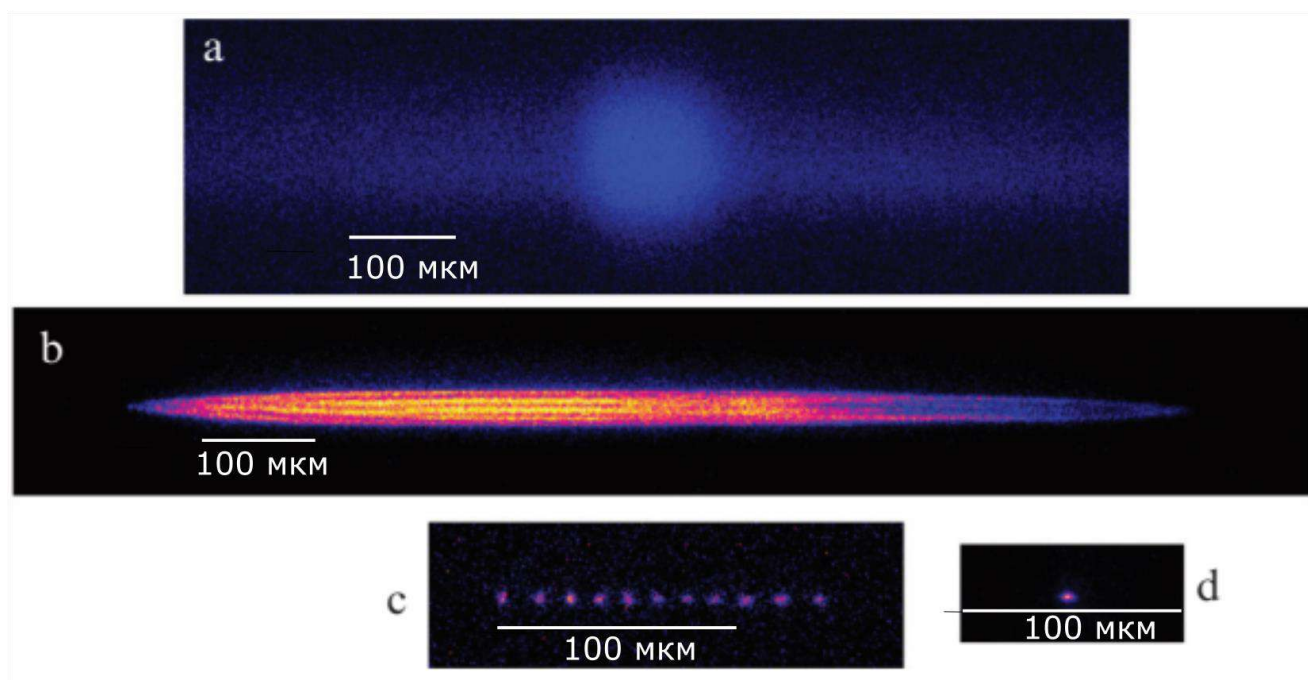
Рис. 28 Изображения различных типов ионных облаков и кристаллов: а – большое облако ионов Mg. В данном случае облако подсвечивалось двумя лазерными пучками: вдоль оси ловушки и ортогонально в плоскости изображения в центре ловушки. Этим объясняется специфичность формы наблюдаемого облака. б – большой ионный кристалл ионов \text{Mg}^+ . Смещение плотности кристалла влево объясняется относительно слабым удерживающим потенциалом вдоль оси
