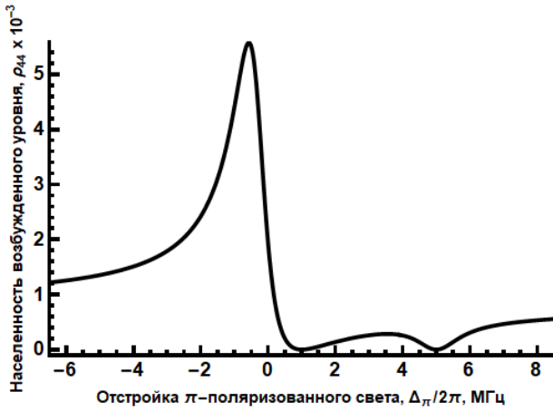
Рис. 36. населенность верхнего уровня от отстройки линейно поляризованного излучения \Omega_{\sigma^-} = 2,5 Г, \Omega_{\sigma^+} = 25 Г, \Omega_{\pi} = 15 Г; \Delta_{\sigma^+} = 2\pi \times 1 МГц, \Delta_{\sigma^-} = 2\pi \times 5 МГц.
