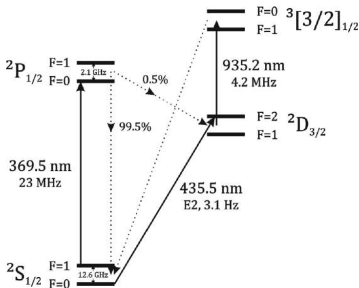
Рис. 33. Структура энергетических уровней ^{171}\text{Yb}^+ используемая в работе.
