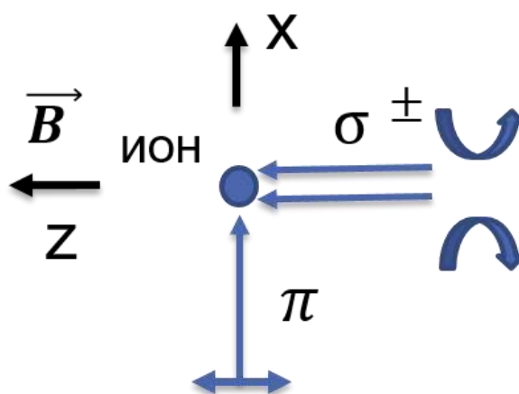
Рис. 35 Схема лазерных пучков, участвующих в методе охлаждения при помощи двойной индуцированной прозрачности.
