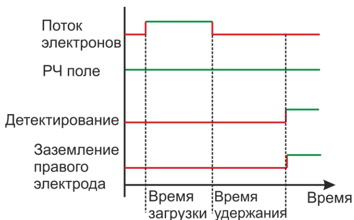
Рис. 23 Временная последовательность в экспериментах по загрузке и времени жизни ионов в линейной квадрупольной ловушке Пауля. Зеленым показано включенное состояние, красным - выключенное
