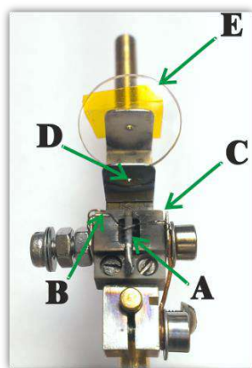
Рис. 13 атомный испаритель на основе танталовой трубки. А – танталовая трубка, В – нагревательная проволока, С – керамический изолятор, D – диафрагма, E – покровное стекло для тестирования работы атомного испарителя
