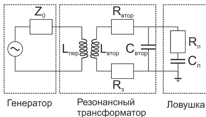
Рис. 16. Эквивалентная схема резонансного трансформатора. Z_0 – импеданс генератора, R_{\text{втор}} – сопротивление вторичной катушки резонансного трансформатора, R_3 – активное сопротивление заземления резонансного трансформатора R_{\text{л}} – активное сопротивление электродов ловушки, C_{\text{л}} – емкость электродов ловушки, C_{\text{втор}} – емкость вторичной катушки резонансного трансформатора, L_{\text{пер}} – индуктивность первичной катушки, L_{\text{втор}} – индуктивность вторичной катушки
